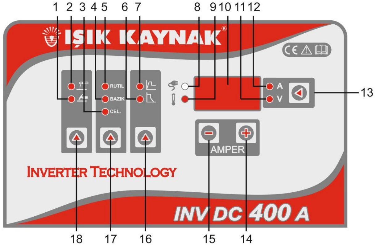
Şekil 3: Kontrol Paneli
